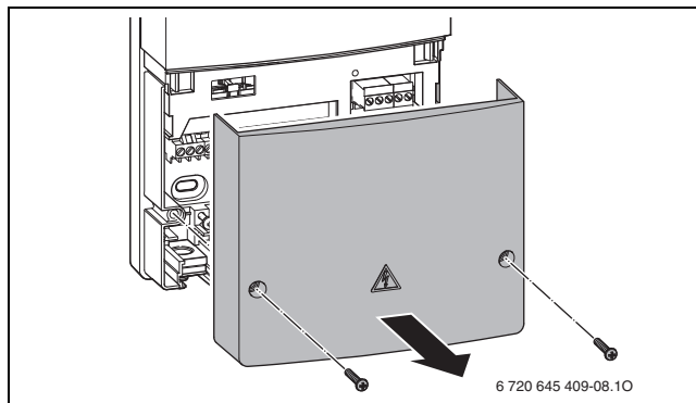
Рис. 39 Откройте корпус
