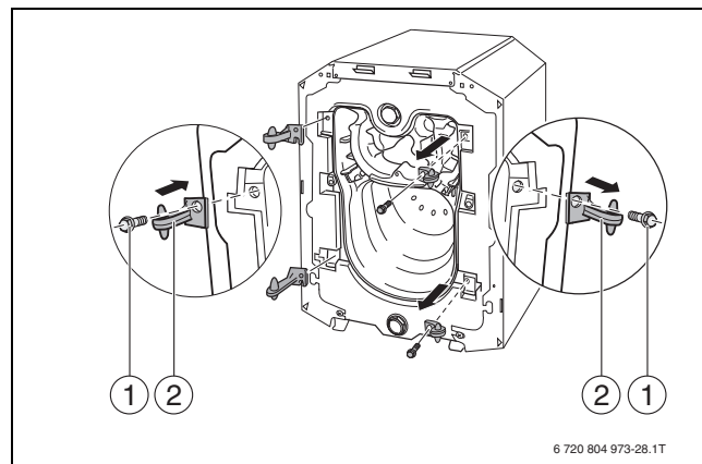
Рис. 14 Переустановка двери топочной камеры (со стороны блока котла)
