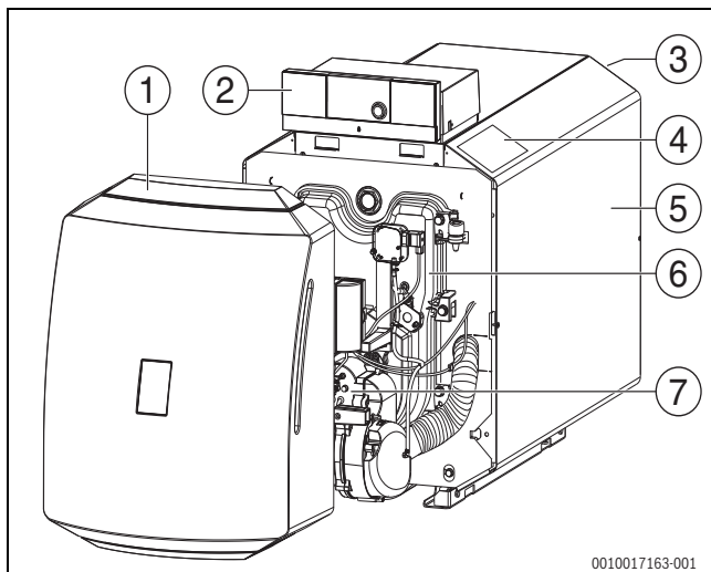
Рис. 1 Вид спереди
