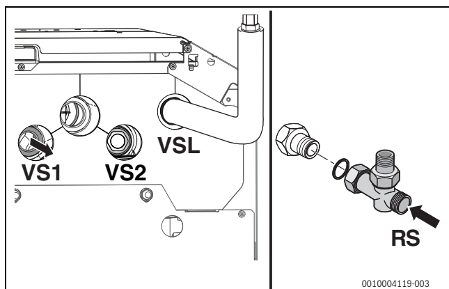
Рис. 30 Подключение бака-водонагревателя
