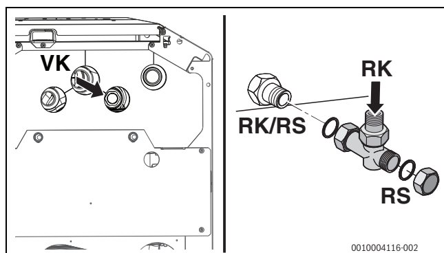
Рис. 27 Подключение подающей и обратной линий
