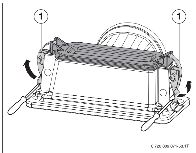
Рис. 76 Открытие быстросъёмных замков
