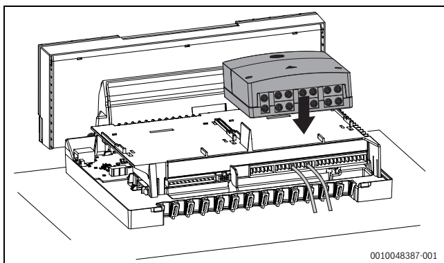
Рис. 42 Установка функциональных модулей
