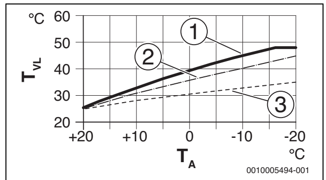
Рис. 65 Настройка отопительной кривой для обогрева пола. Угол наклона определяется расчетной температурой T_{AL} и минимальной наружной температурой T_{A,min}
