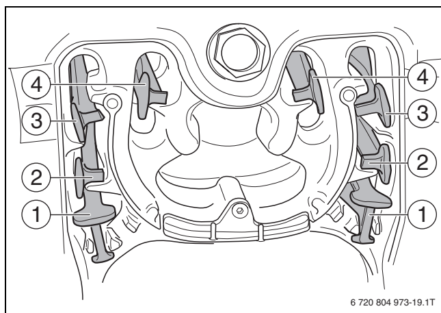
Рис. 46 Направляющие пластины горячих газов 18, 22, 30 и 49 кВт
