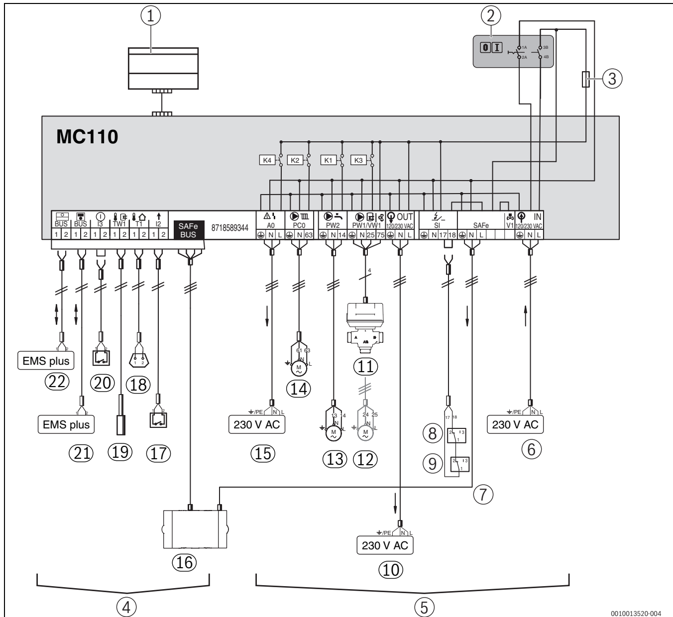
Рис. 89 Схема соединений системы управления MC110
