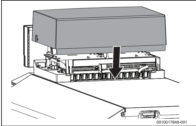
Рис. 44 Установка верхней крышки
