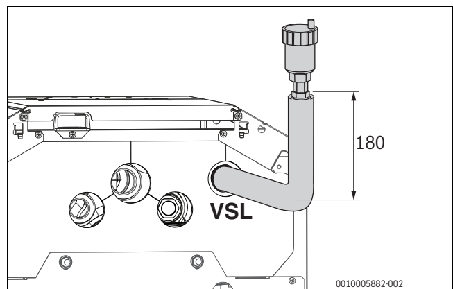
Рис. 28 Подключение воздухоотводчика к предохранительной линии (размеры в мм)
