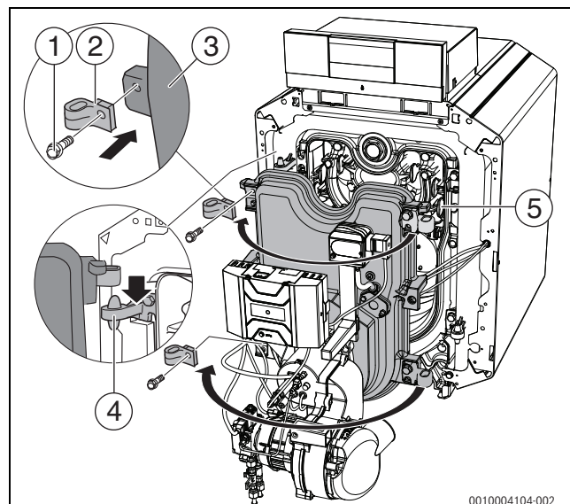
Рис. 15 Переустановка двери топочной камеры (со стороны двери)
