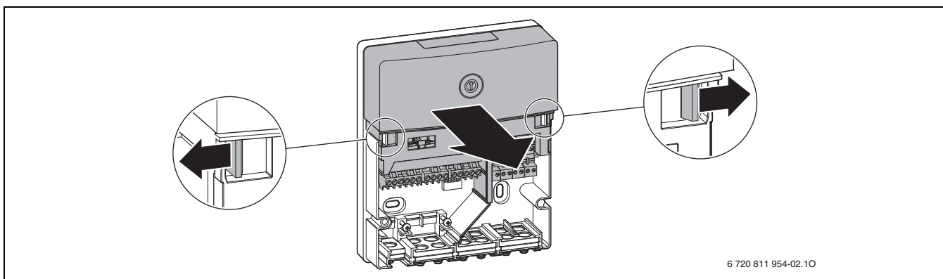
Рис. 40 Удалите функциональный модуль
