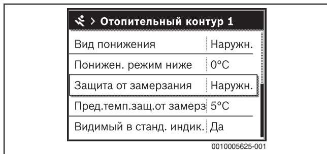
Рис. 59 Применение защиты от замерзания
