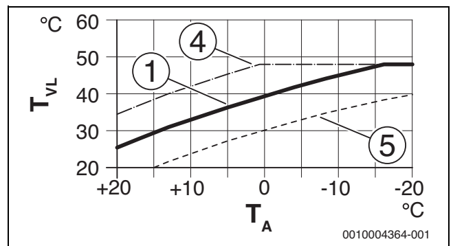
Рис. 66 Настройка отопительной кривой для обогрева пола. Параллельное смещение через Смещение комн. темп. или вследствие изменения требуемой комнатной температуры
