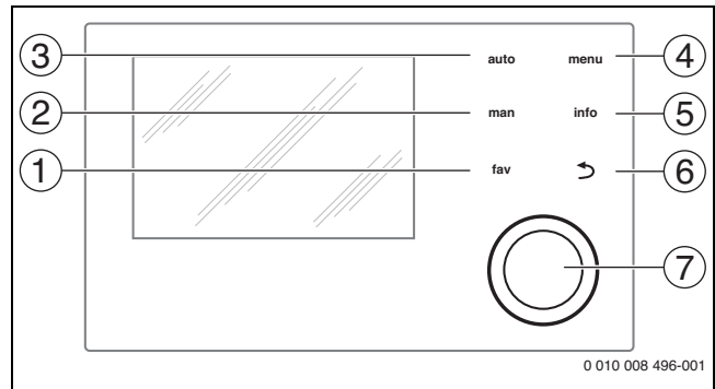
Рис. 52 Элементы управления
