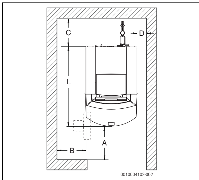
Рис. 13 Расстояния от стен в помещении (вид сверху) (котёл располагается слева или справа)
