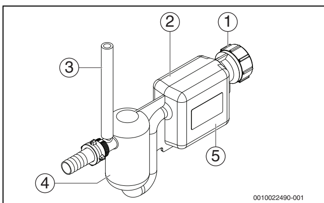
Рис. 23 Сифон, версия 2
