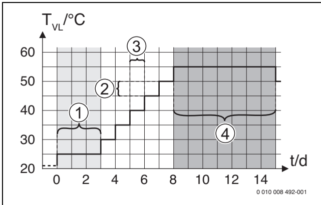
Рис. 69 Выполнение сушки пола с первоначальными установками на стадии нагрева
