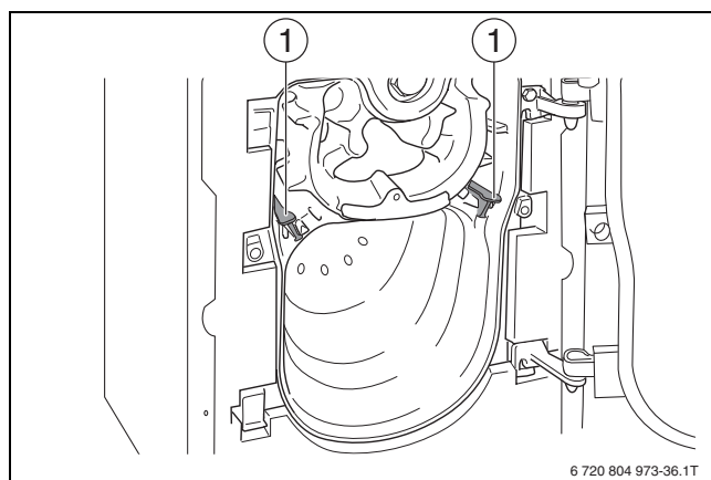
Рис. 71 Открытие двери топочной камеры (например, 35 кВт)
