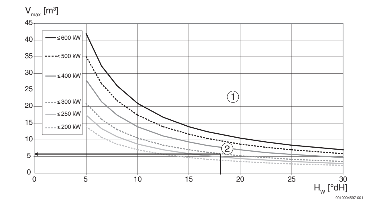
Рис. 88 Требования к воде для заполнения и подпитки теплогенераторов из чёрных металлов (чугуна и нелегированных сталей) мощностью от 200 до 600 кВт
