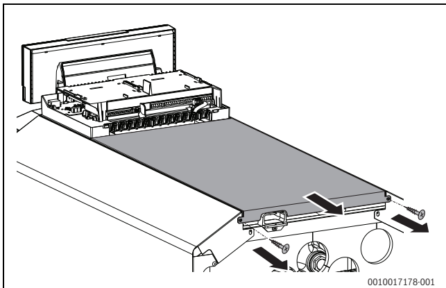
Рис. 36 Открывание задней крышки
