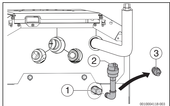
Рис. 29 Подключение комплекта для удаления воздуха
