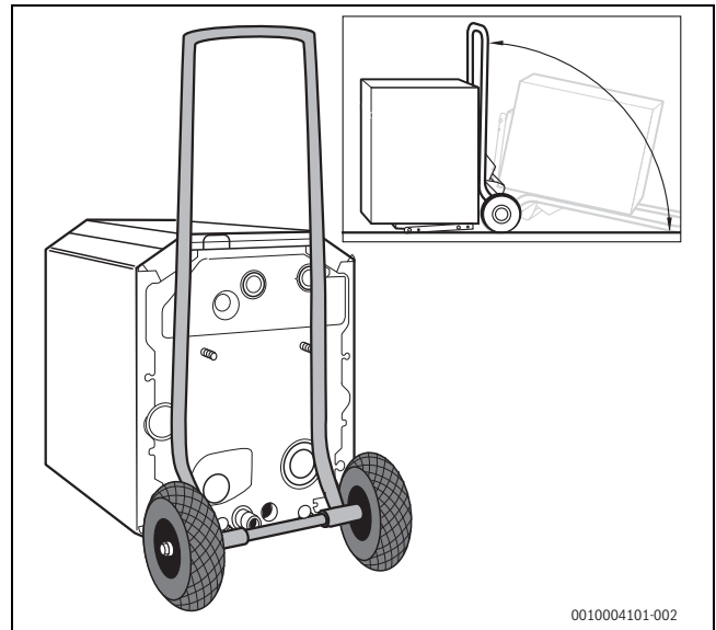
Рис. 12 Перевозка котла на тележке
