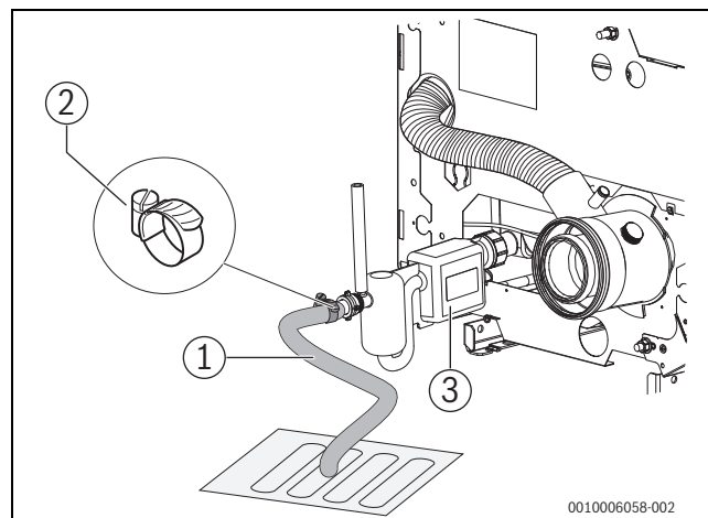
Рис. 24 Конденсатоотвод без нейтрализации конденсата, показан сифоном версии 2
