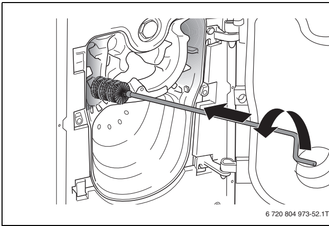
Рис. 72 Чистка газоотводящих каналов щёткой
