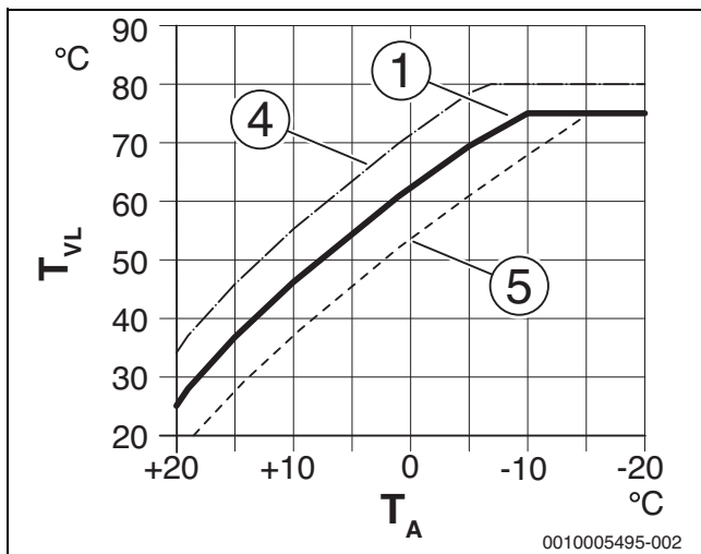
Рис. 68 Настройка отопительной кривой для радиаторов Параллельное смещение через Смещение комн. темп. или вследствие изменения требуемой комнатной температуры
