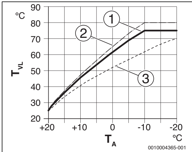
Рис. 67 Настройка отопительной кривой для радиаторов Угол наклона определяется расчетной температурой T_{AL} и минимальной наружной температурой T_{A,min}
