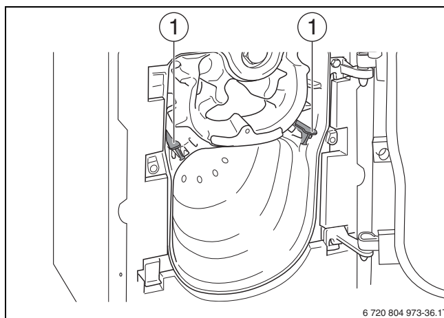
Рис. 47 Направляющие пластины горячих газов 35 кВт
