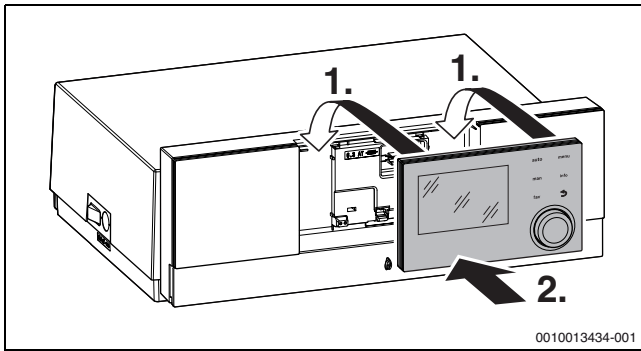
Рис. 50 Установка пульта управления
