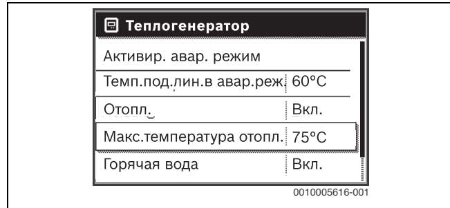
Рис. 57 Максимальная температура подающей линии
