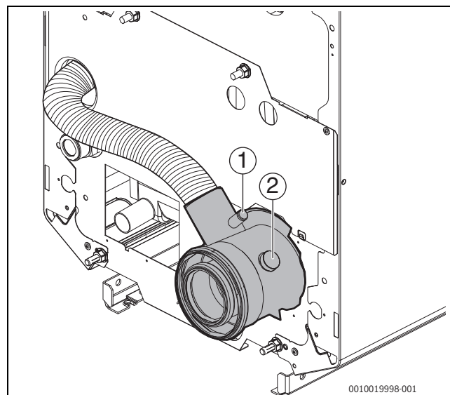
Рис. 5 Соединительный штуцер концентрической дымовой трубы
