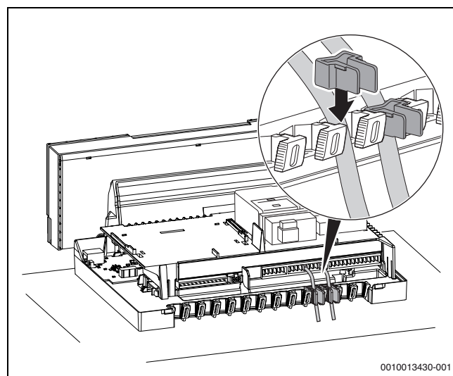
Рис. 43 Клеммная колодка на системе управления
