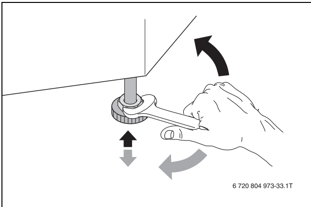
Рис. 19 Горизонтальное выравнивание котла
