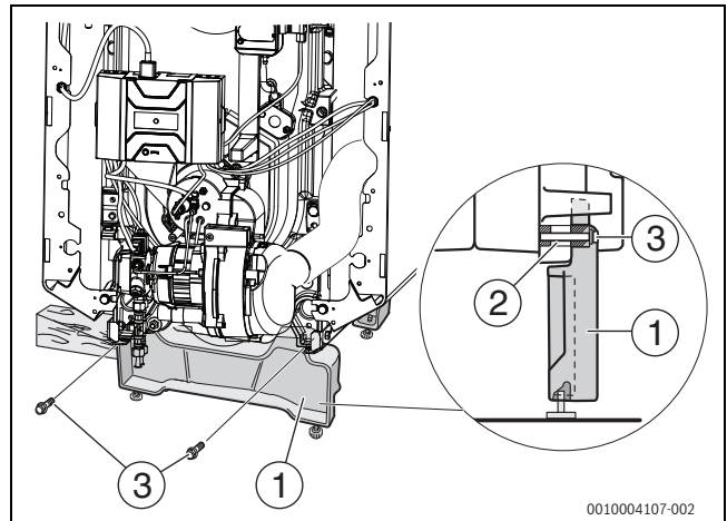
Рис. 18 Монтаж цоколя на переднем элементе
