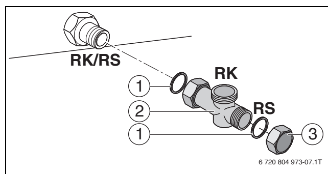
Рис. 25 Монтаж тройника обратной линии
