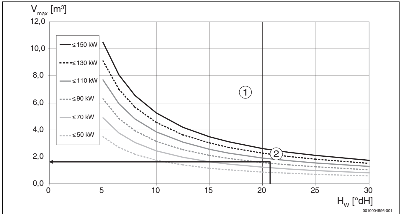
Рис. 87 Требования к воде для заполнения и подпитки теплогенераторов из чёрных металлов (чугуна и нелегированных сталей) мощностью до 150 кВт
