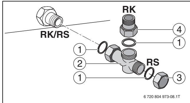
Рис. 26 Монтаж тройника обратной линии
