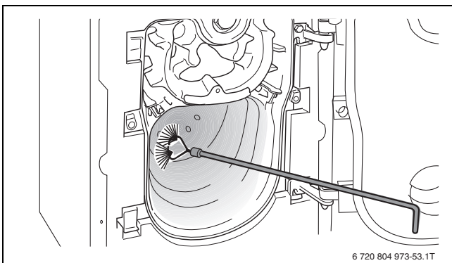
Рис. 73 Чистка щёткой камеры сгорания
