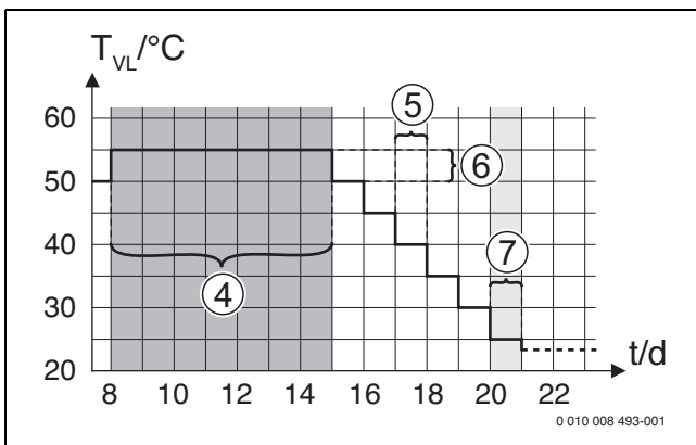
Рис. 70 Выполнение сушки пола с первоначальными установками на стадии охлаждения
