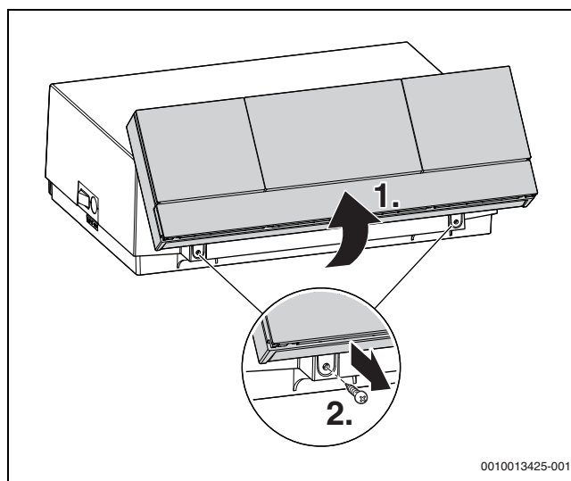
Рис. 34 Пульт управления откинут вверх
