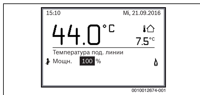
Рис. 60 Режим "Тест дымовых газов" активирован
