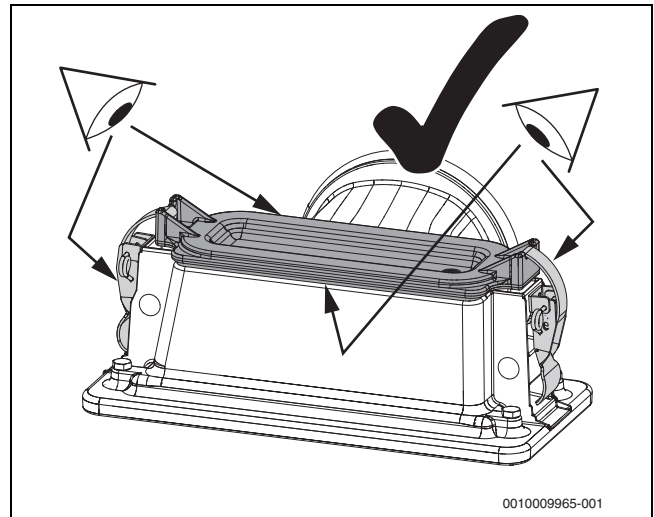
Рис. 80 Проверка правильной посадки крышки люка для чистки и быстросъёмных замков
