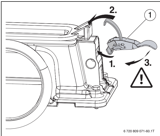
Рис. 78 Установка быстросъёмных замков
