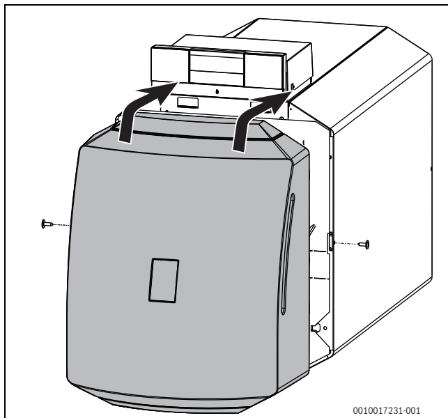
Рис. 62 Установка кожуха горелки
