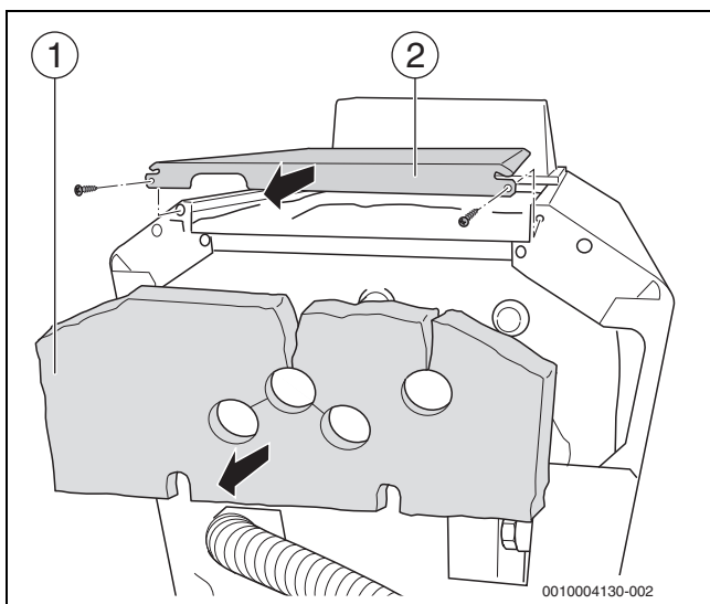
Рис. 74 Откройте экономайзер
