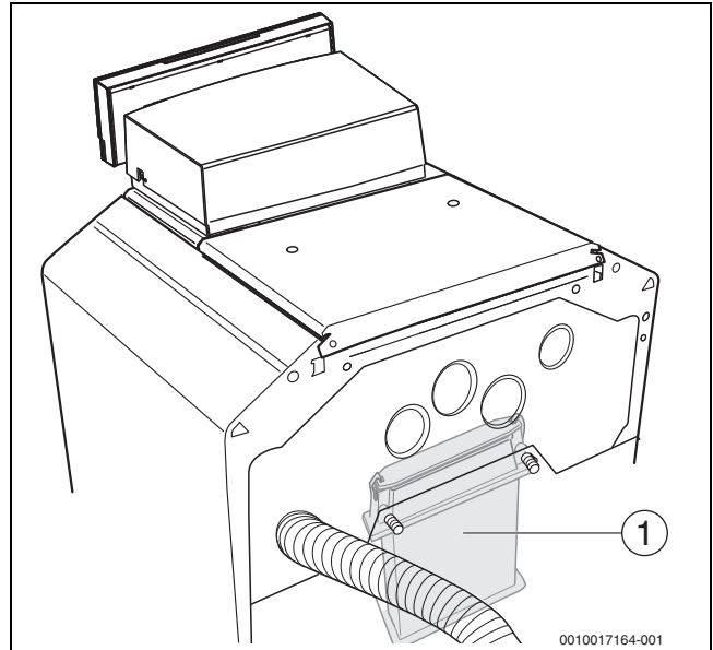
Рис. 2 Вид сзади (показано без теплоизоляции)
