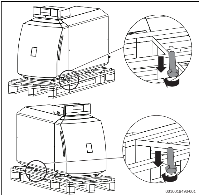
Рис. 6 Удаление транспортного фиксатора (для котла 60 кВт)
