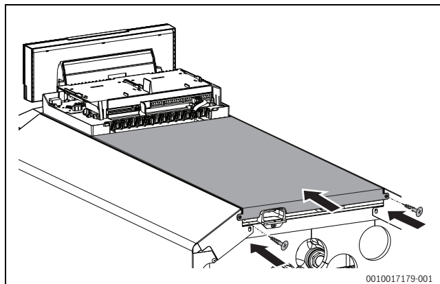
Рис. 37 Монтаж крышки
