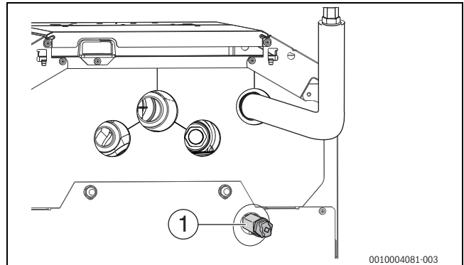
Рис. 33 Удаление воздуха из теплообменника
