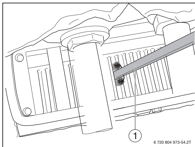
Рис. 77 Чистка экономайзера щёткой (вид сверху)
