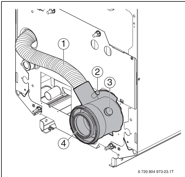
Рис. 20 Монтаж штуцера подачи воздуха - отвода дымовых газов
