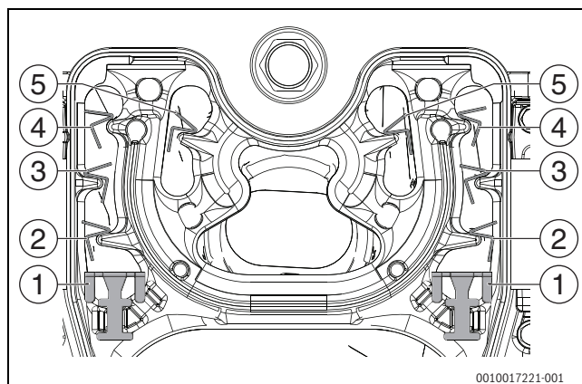
Рис. 48 Направляющие пластины горячих газов 60 кВт
