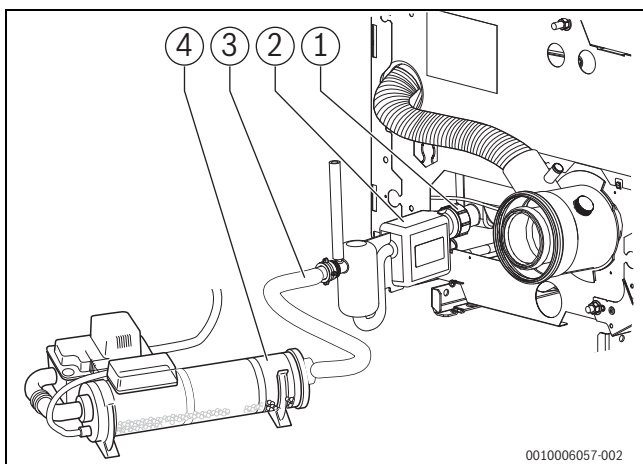
Рис. 22 Конденсатоотвод с нейтрализацией
