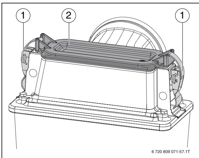
Рис. 75 Теплообменник
