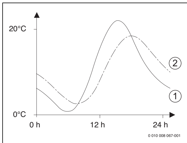
Рис. 64 Пример демпфированной наружной температуры
