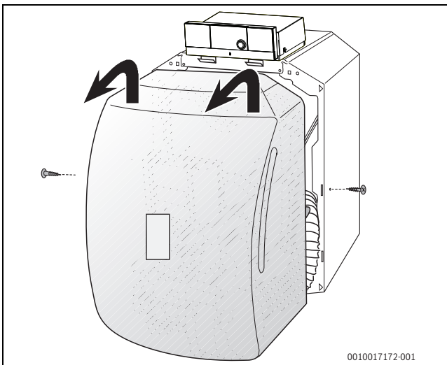
Рис. 7 Демонтаж кожуха горелки
