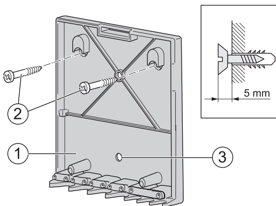
Рис. 8 Установка настенного кронштейна
