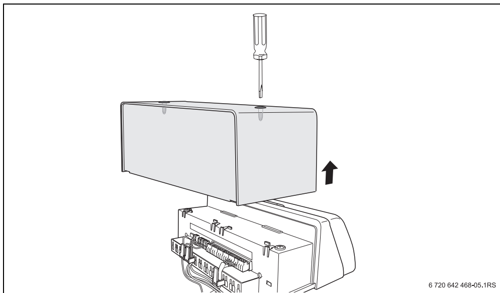
Рис. 4 Снятие верхней крышки
