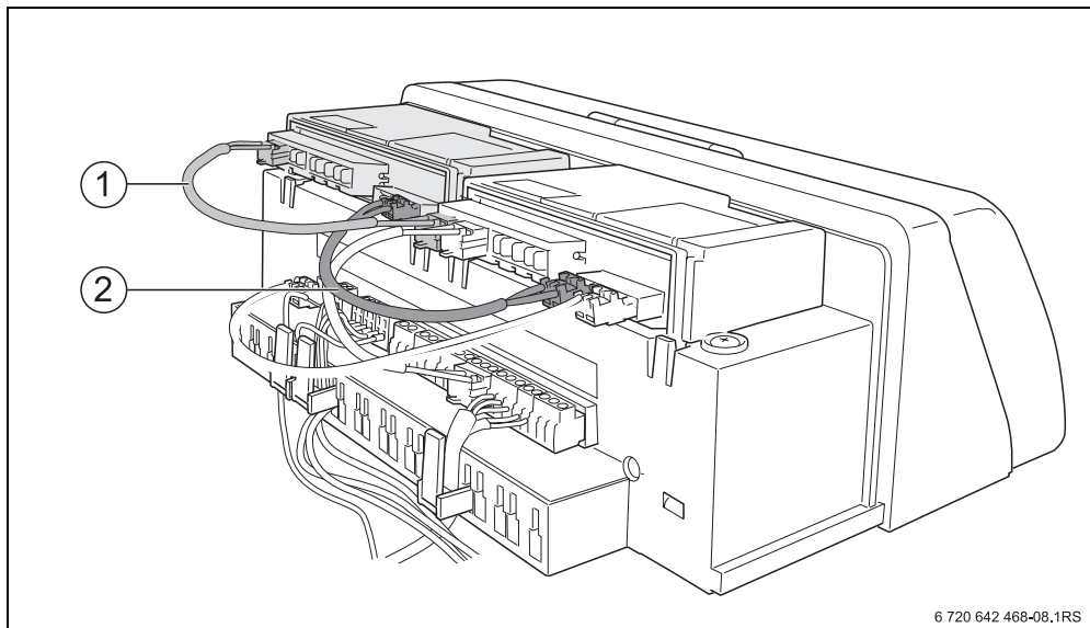
Рис. 7 Подключение второго функционального модуля xM10
