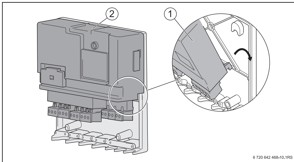
Рис. 9 Установка функционального модуля
