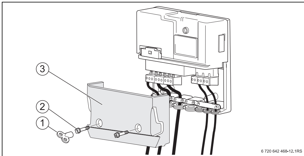
Рис. 11 Установка клеммной крышки
