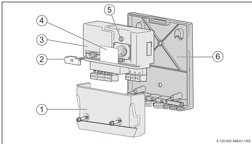
Рис. 1 Функциональный модуль (здесь: настенный монтаж)
