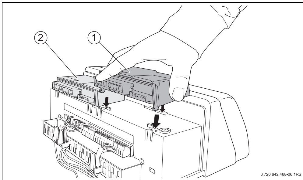
Рис. 5 Установка функционального модуля
