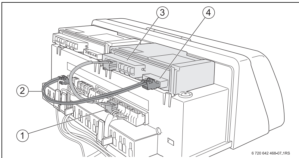
Рис. 6 Подключение первого функционального модуля
