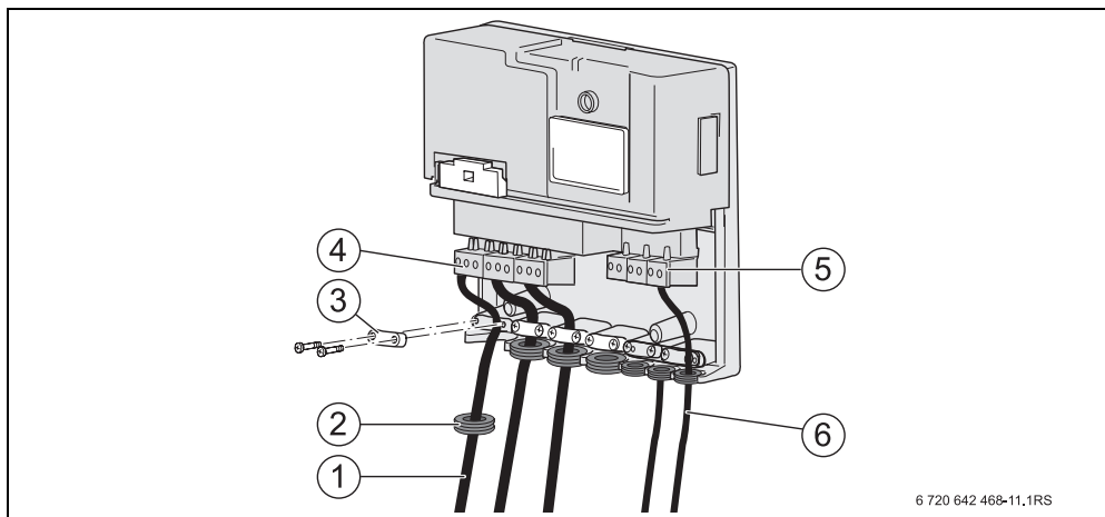
Рис. 10 Выполнение электрических подключений
