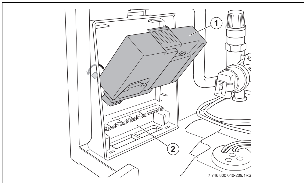
Рис. 2 Установка функционального модуля
