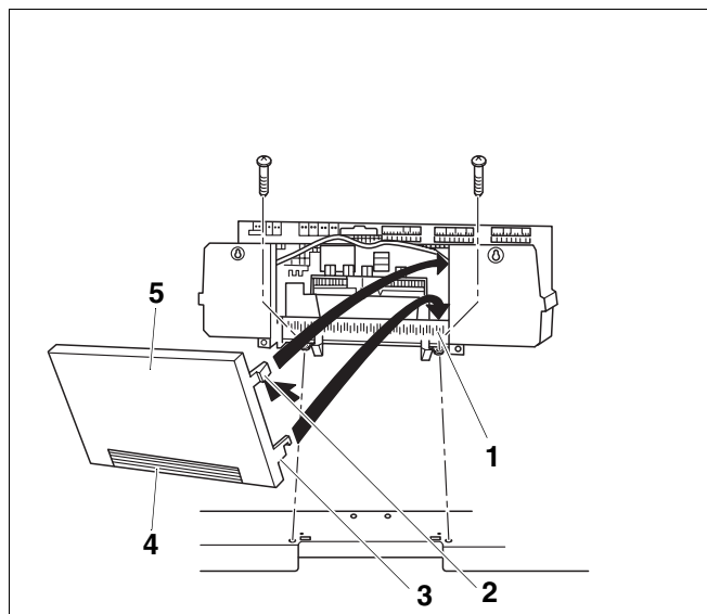
Рис. 67 Установка задней стенки системы управления
