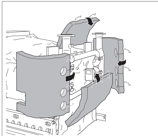
Рис. 51 Укладка теплоизоляции на трубы
