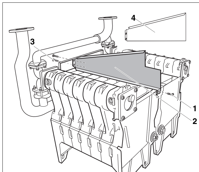
Рис. 36 Установка перегородки
