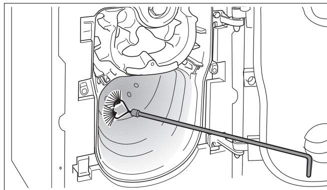
Рис. 45 Чистка топочной камеры
