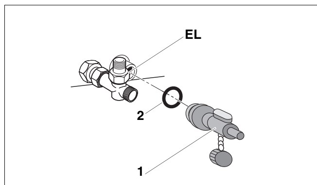
Рис. 24 Установка крана для наполнения и слива
