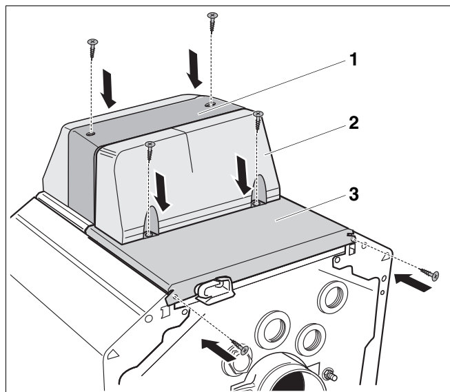
Рис. 30 Установка крышек
