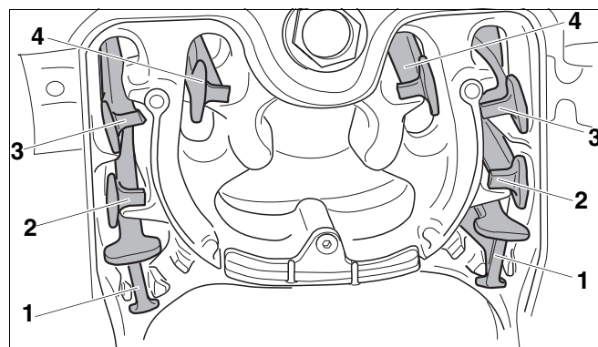
Рис. 37 Направляющие пластины дымовых газов отопительного котла, работающего с забором наружного воздуха на горение
