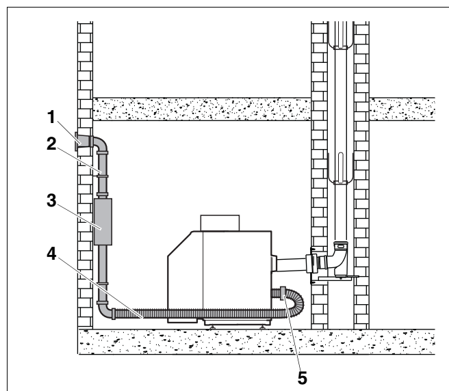
Рис. 18 Система подачи воздуха на горение и отвода дымовых газов (пример для вида монтажа OC 53x )
