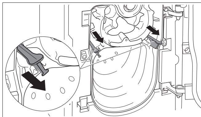
Рис. 36 Удаление направляющих пластин дымовых газов
