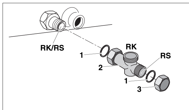
Рис. 19 Монтаж соединительного элемента обратной линии
