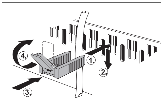
Рис. 29 Крепление проводов хомутами
