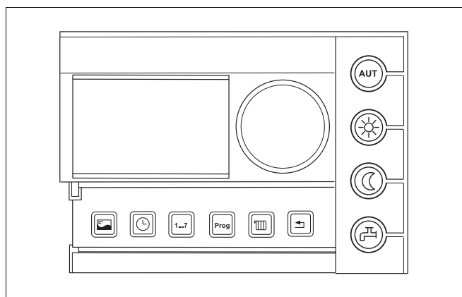
Рис. 40 Пульт управления (например, RC30 с открытой крышкой)
