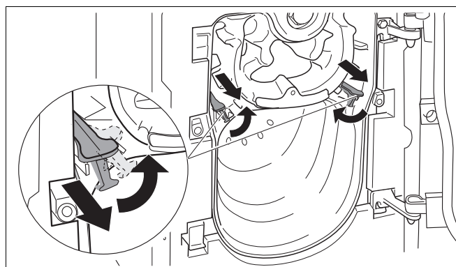
Рис. 35 Перестановка направляющих пластин дымовых газов
