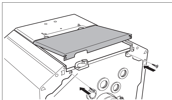
Рис. 26 Снятие задней крышки котла
