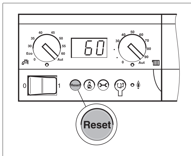
Рис. 47 Сброс неисправности нажатием кнопки "Reset"
