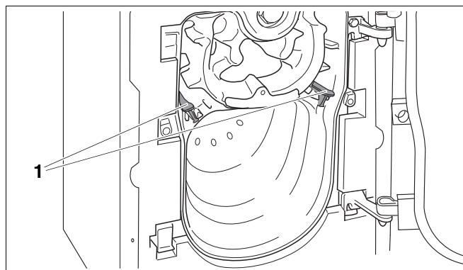
Рис. 43 Открытая дверца горелки
