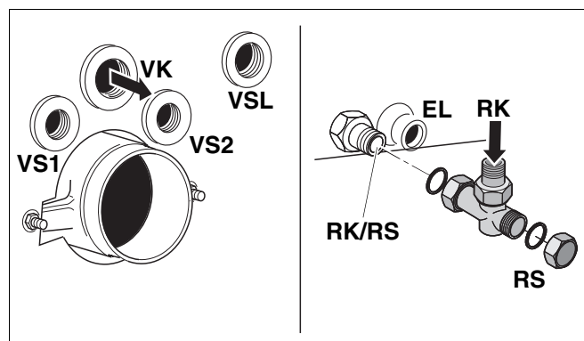
Рис. 21 Подключение подающей и обратной линий
