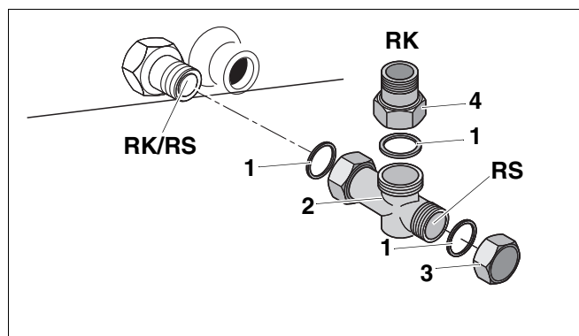
Рис. 20 Монтаж соединительного элемента обратной линии
