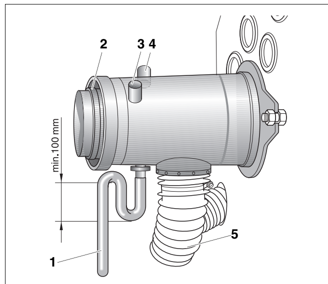
Рис. 17 Монтаж присоединительного концентрического штуцера
