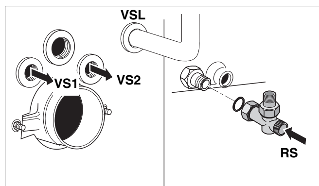
Рис. 23 Подключение бака-водонагревателя
