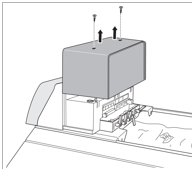
Рис. 28 Снятие верхней крышки
