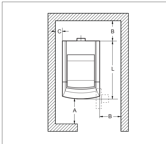
Рис. 8 Расстояния от стен в помещении (котел располагается справа или слева от входа)
