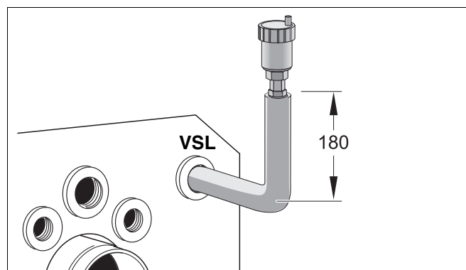
Рис. 22 Подключение воздушного клапана к предохранительной линии (размеры в мм)
