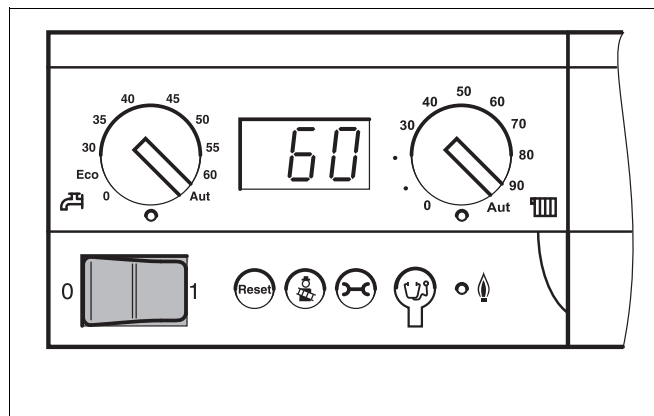
Рис. 42 Включение отопительной установки
