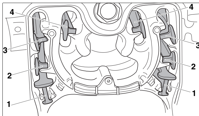
Рис. 33 Направляющие пластины дымовых газов отопительного котла, работающего с забором наружного воздуха на горение
